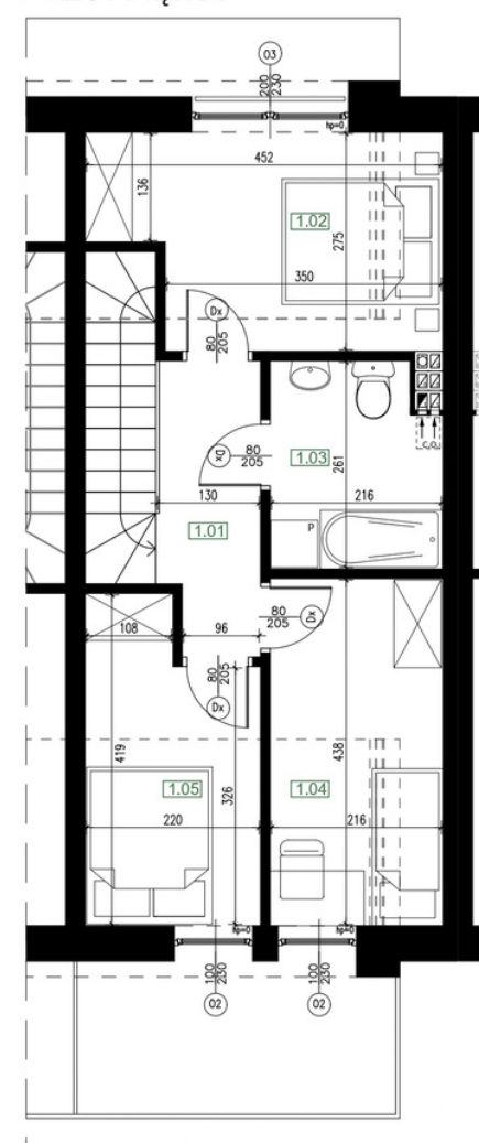
RZUT PIĘTRA
